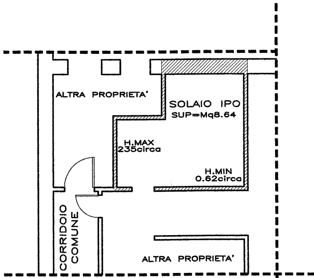
SOLAIO PIANO SESTO SCALA 1:100
