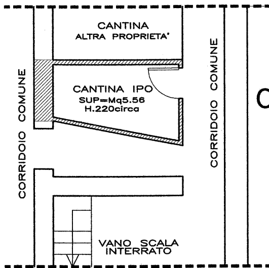
CANTINA PIANO INTERRATO SCALA 1:100
